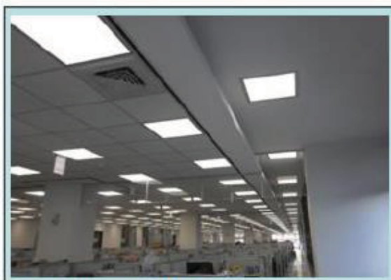
迴路ON時照度1110 lux
